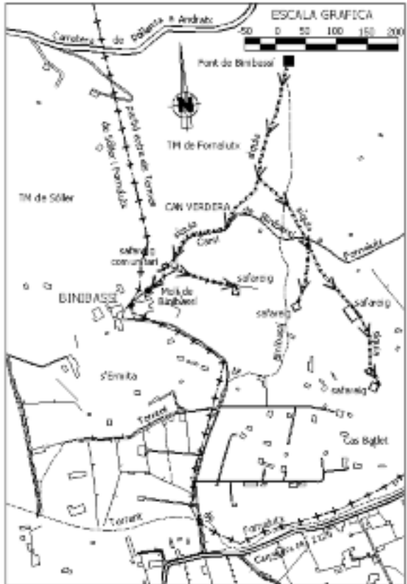
Plànol 2.- Font i síquia de Binibassí fins al molí (Topògraf: Josep Ll. Sunyer).
