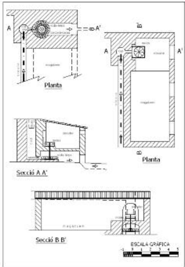
Plànol 1.- Esquema del molí de Monnàber (Topògraf: Josep Ll. Sunyer).
