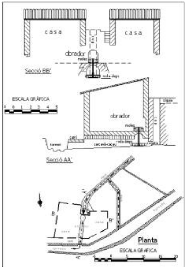
Plànol 7.- Esquema del Molí d'Amunt (Topògraf: Josep Ll. Sunyer).
