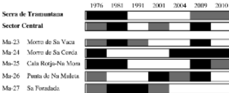
Fig. 4. Tendència de la població de la Serra de Tramuntana, la del sector central i de cadascuna de les colònies que formen el sector central expressada en la metodologia de Traffic Lights , significat dolent el negre, intermedi el gris i bo el blanc.
