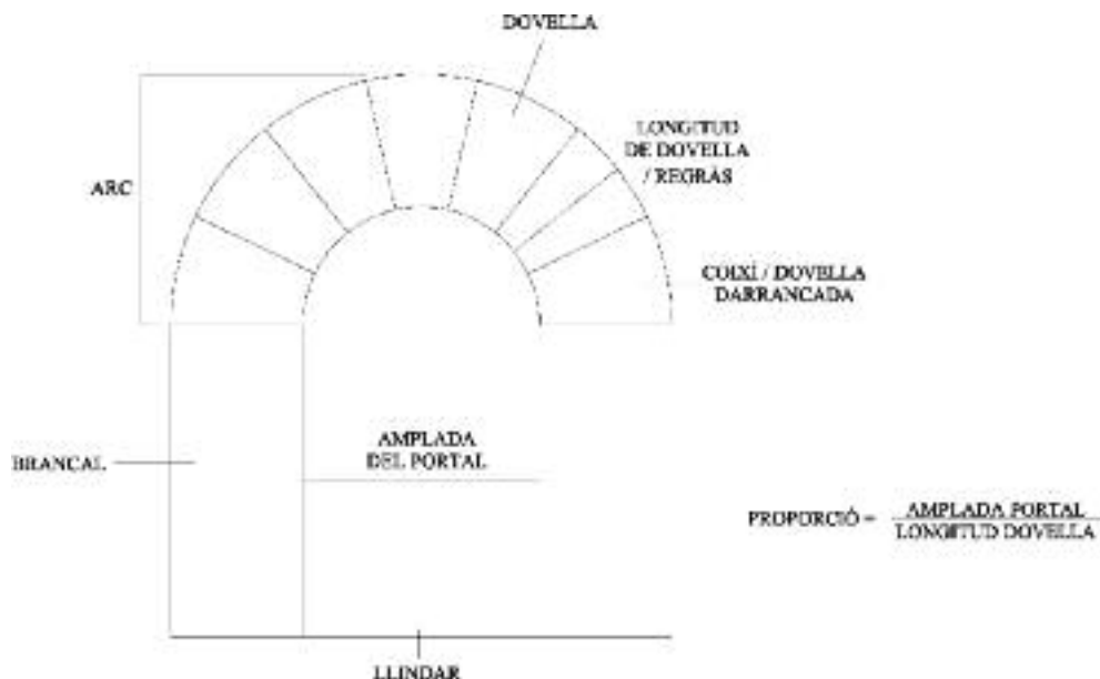
Esquema de les parts d'un portal rodó.
