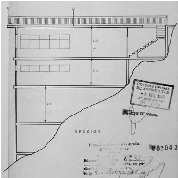
Figura 7 Secció de la tercera ampliació de l'edifici del Mirador de Ses Barques, Antonio Parietí, 1970. Arxiu Municipal de Sóller, fons llicències d'obra, expedient núm 19/1970.
