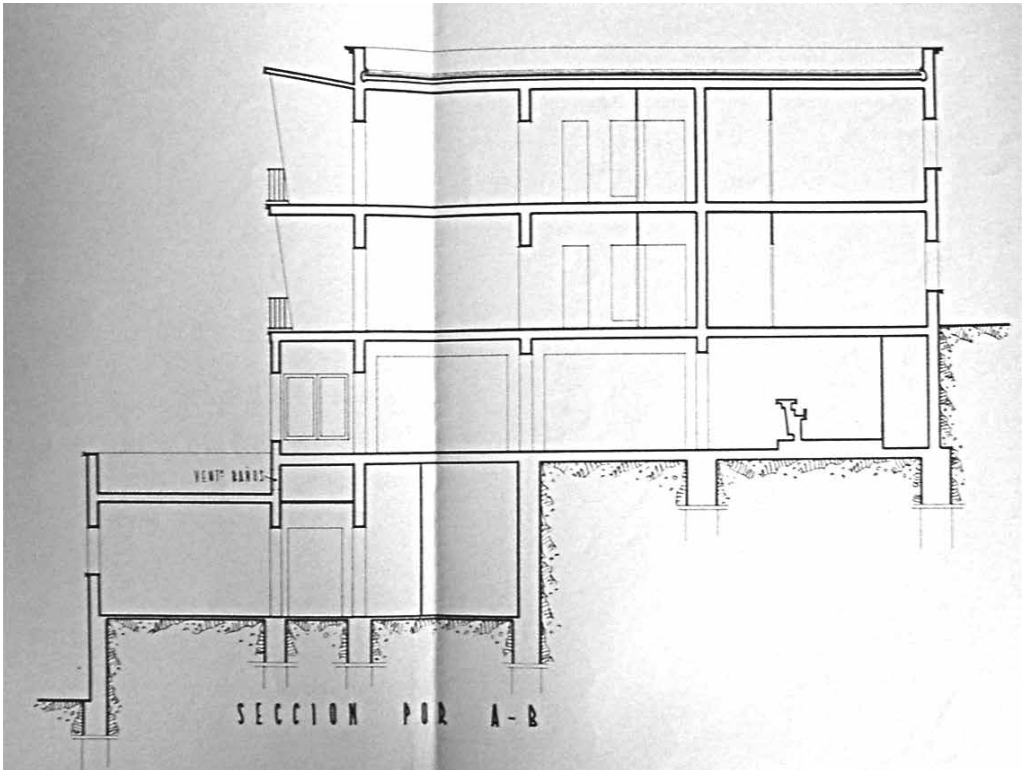
Figura 5 Secció de l'hotel Marbell. Antoni Coll, 1959. Arxiu Municipal de Sóller, fons llicències d'obra, expedient núm. 25/1959.
