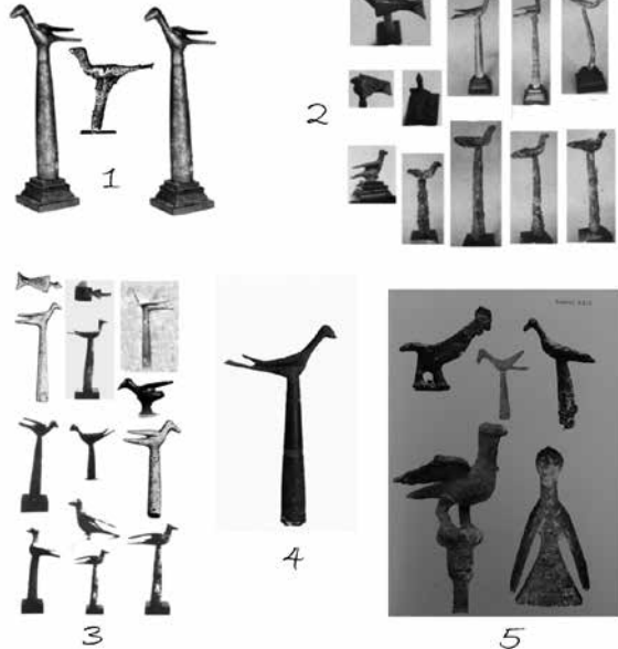
Colometes localitzades a Mallorca: Son Taixaquet (1), Cova Monja (2), Son Cresta (3), Son Ribot (4) i Cometa des Mortis (5).
