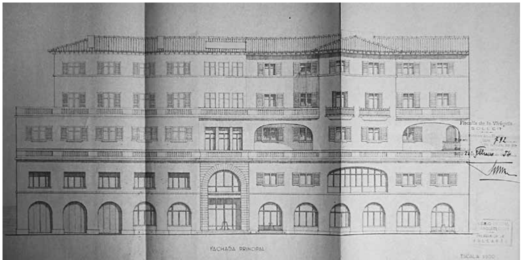
Figura 4 Façana principal de l'hotel Espléndido, Antoni Coll i Rafael Pomar, 1954. Arxiu Municipal de Sóller, fons llicències d'obra.
