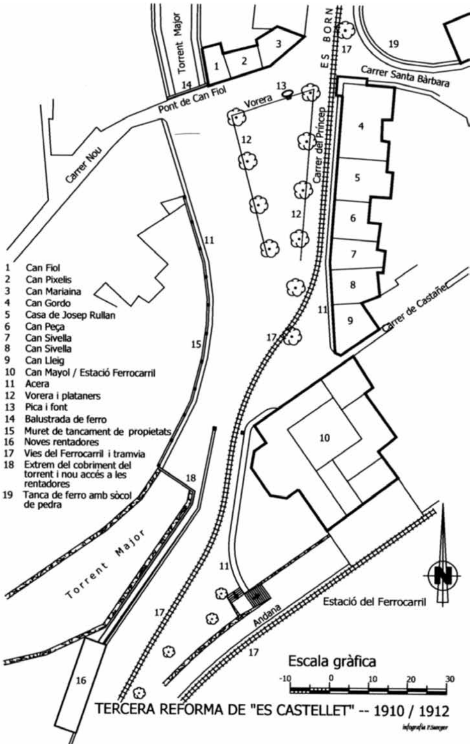
Plànol de la zona del Castellet després de la reforma de 1911-1913. Elaboració: Antoni Quetglas i Josep Sunyer
