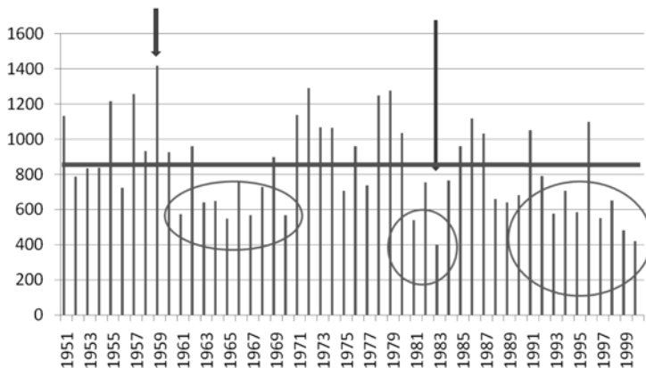
Figura 2. Totals anuals (mm) de precipitació a l'estació B061.
