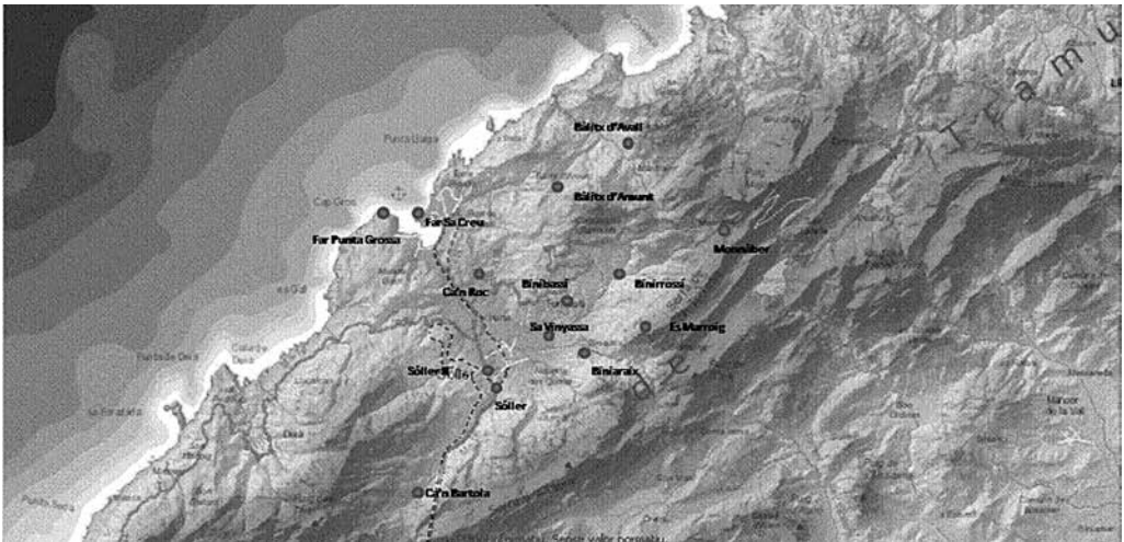
Figura 1. Situació de les estacions meteorològiques. Font: Elaboració pròpia.
