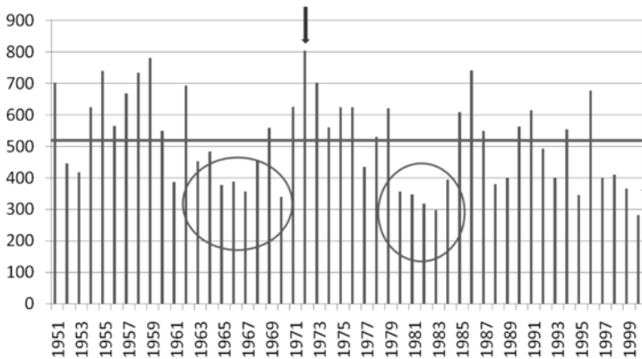
Figura 3. Totals anuals (mm) de precipitació a l'estació B075.
