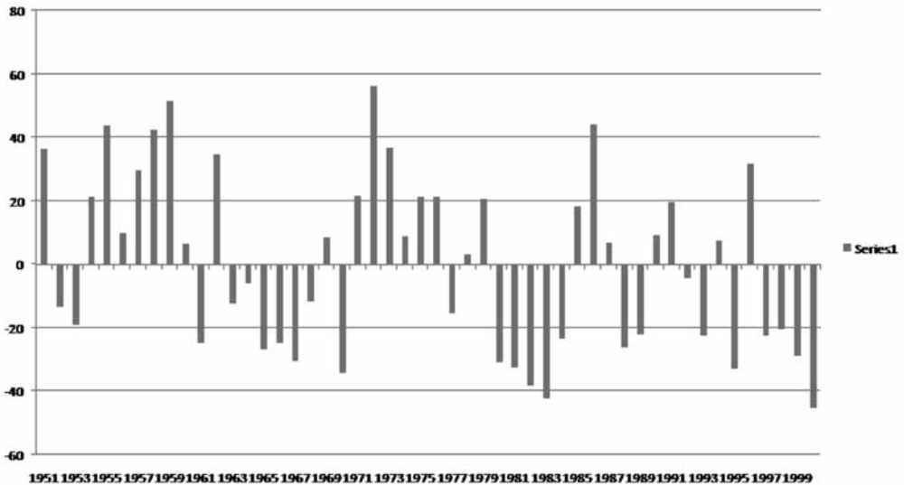
Figura 5. Anomalies pluviométriques anuals a l'estació B075 Far Punta Grossa.
