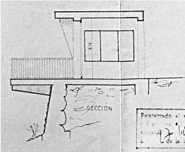
Figura 7 Secció de la tercera ampliació de l'edifici del Mirador de Ses Barques, Antonio Parietí, 1970. Arxiu Municipal de Sóller, fons llicències d'obra, expedient núm 19/1970.
