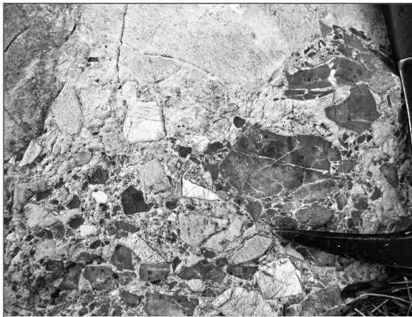
Fig. 18 Bretxes polimíctiques a la zona de Muleta. S'observen diferents tipus de clastes de diferents coloracions i amb matriu de coloració clara, gairebé blanca. Els clastes són molt angulars i indiquen un transport cap al lloc de compactació gairebé immediat. En aquest cas es donaria el mateix resultat a partir de la hipòtesi del talús o de la de l'impacte.
