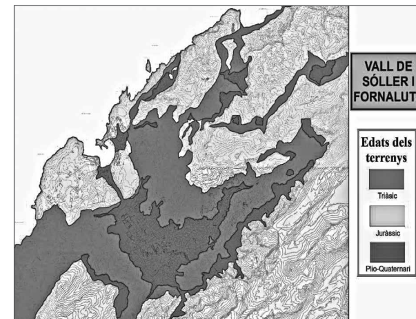
Fig. 7 Mapa geològic sintètic i simplificat de la Vall de Sóller i Fornalutx (no mostra materials del Miocè inferior)
