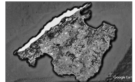
Fig. 15 Distribució aproximada de les bretxes a la Serra de Tramuntana.
