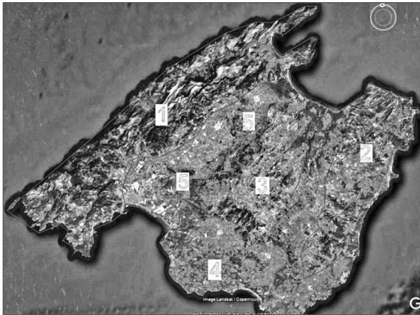
Fig. 6 Les 5 zones geològiques de Mallorca
