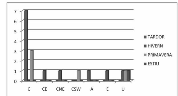
Figura 3. Repartiment mensual de les situacions sinòptiques.
