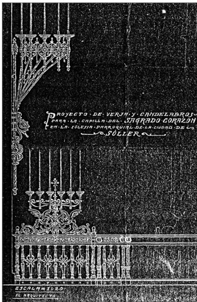
Disseny del reixat de ferro de la capella del Cor de Jesús obra de Joan Rubió. El feren els ferrers Josep Bauzá i el seu cosí Damià Bauzá.
