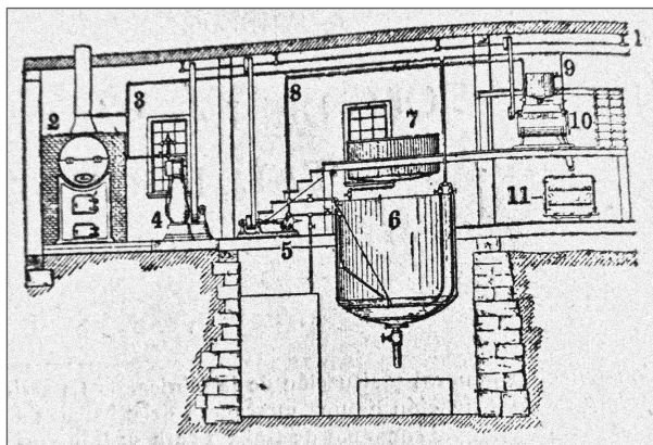
Funcionament de la fàbrica de sabó. Los métodos más modernos de fabricación de jabones, bujías y glicerinas
