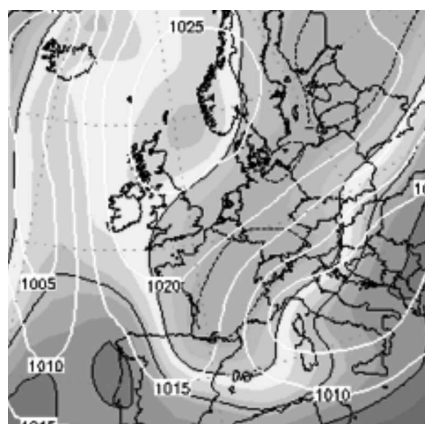
Mapa corresponent a les temperatures que es donaren el 8 d'Octubre de 1936 a una altura de 1500 m. La isoterma dels 0°C va arribar a superar Mallorca, fent així la seva aparició més primerenca coneguda. Font: NCEP.
