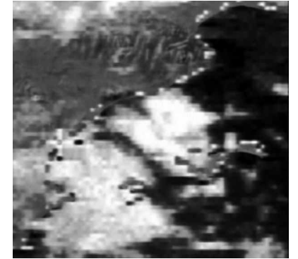
Imatge de satèl·lit corresponent a l'horabaixa de l'1 de Novembre de 1992, on es poden apreciar tots els níguls que amollaven aigua especialment al Nord-Oest de Mallorca. Font: Aemet.
