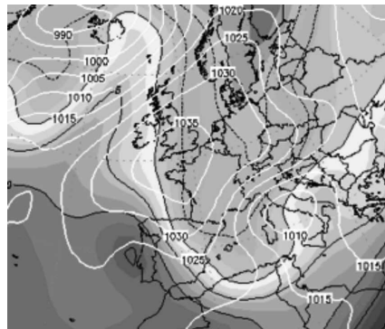
Entre els dies 25 i 26 d'Octubre de 1887 es va produir el rècord temporal d'aproximació de la isoterma dels -4°C/-5°C a 850hpa. Mai més ens ha tornat a visitar tan prest aquesta isoterma. Font: NCEP.
