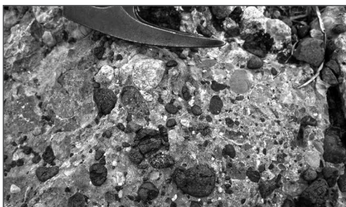
Fig. 11 Pudinga del Miocè de Bàltx d'Amunt. S'observen clastes obscurs de roca volcànica (basalts) i clastes grisos més clars de calcàries juràssiques, amb poca matriu de color blau-grisa
