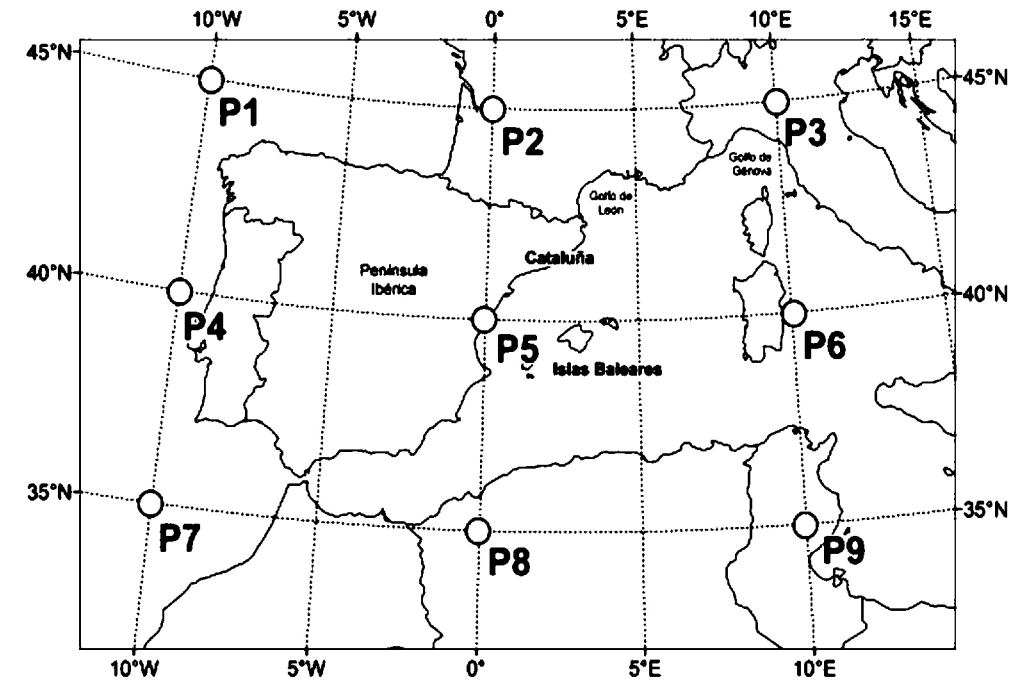
Figura 1. Retícula dels punts d'aplicació de les variables del mètode de Jenkinson i Collison. Font: Llop i Alomar (2012b).
