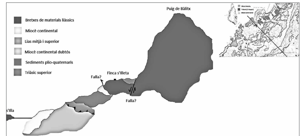
Fig. 9. Tall geològic interpretatiu de l'estructura de la zona de S'Illeta-Puig de Bàltx confeccionat a partir de la cartografia de detall de la zona S'Illeta-Puig de Bàltx
