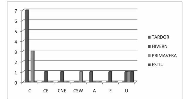
Figura 2. Repartiment estacional de les situacions sinòptiques.
