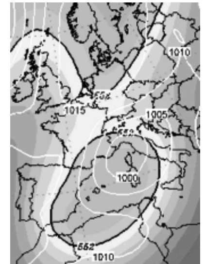
Mapa isobàric on es pot comprovar el gir dels vents cap a Ponent durant la nevada del 22 d'Octubre de 1935. La temperatura baixà fins a -1°C a 1400 metres d'altura. Font: NCEP.
