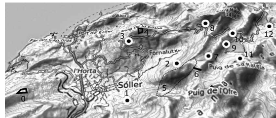
Fig.2. 0.Fortificació puig des Moro. 1.Cova des Negret. 2. Es Xaragall. 3.Cova des Tínel Petit i des Batlet. 4.Puig de sa Bassa. 5.Àrea de refugis des Barranc-Ses Solanes. 6. Fortificació des camins Nous. 7. Cova de sa Bassa i de Son Torrella. 8.Balms des puig des Migdia. 9. Fortificacions del forn de calç. 10. Coval Simó i cova des Penó. 11. Cova de na Franquesa. 12. Almallutx.
