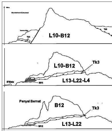
Fig. 10 Talls geològics successius interpretatius de l'estructura de la zona de s'Illeta confeccionat a partir de la cartografia de detall de la zona s'Illeta-Puig de Bàltx-Ses Bases del Bisbe-sa Figuera. A la figura de dalt, falla espectacular prop de la finca de s'Illeta, que indica unes caigudes per gravetat de la zona de sa Font des Joncar
