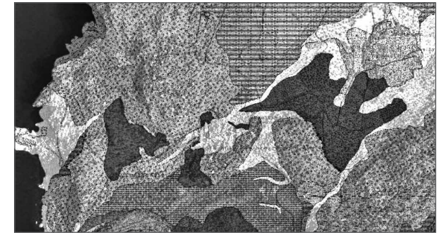
Fig. 8. Mapa geològic confeccionat a partir de la cartografia de detall de la zona d'Alconàsser-Es Gall-Muleta.
