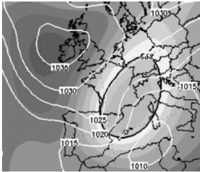
Mapa isobàric corresponent a la nit del 24 d'Octubre de 1941. Font: NCEP.
