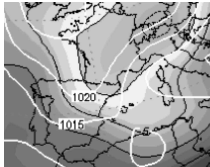
Mapa d'isotermes corresponent al matí del 30 de Setembre de 1936. La isoterma de +2°C a 1500 metres d'altura va tocar l'arxipèlag; és el valor més baix que hem tengut mai dins un mes de Setembre. Font: NCEP.
