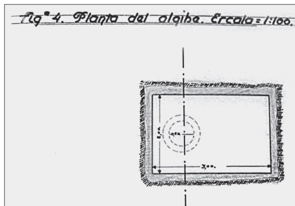
Plànols de l'aljub de Ca Madó Pilla (Valldemossa). Un aljub idèntic al de la Mola de Tuent.
