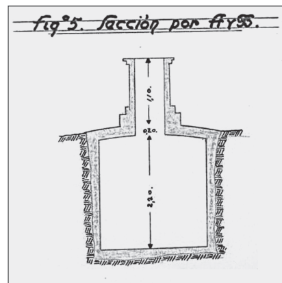
Plànols de l'aljub de Ca Madó Pilla (Valldemossa). Un aljub idèntic al de la Mola de Tuent.
