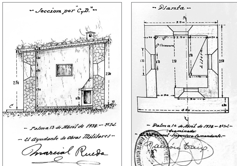
Els plànols de la façana principal, la lateral, la secció per C i D i el de la planta (CHCMBAL).
